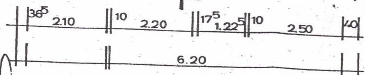
GRUNDRISS M 1:100
